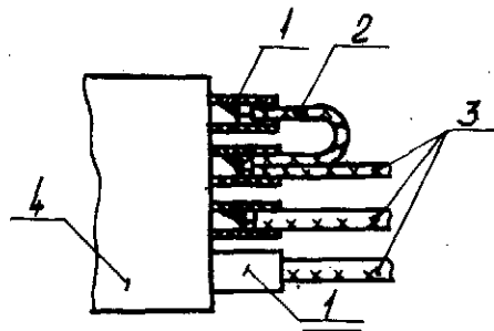
1 - трубка изоляционная; 2 - перемычка; 3 - провода; 4 - корпус соединителя
