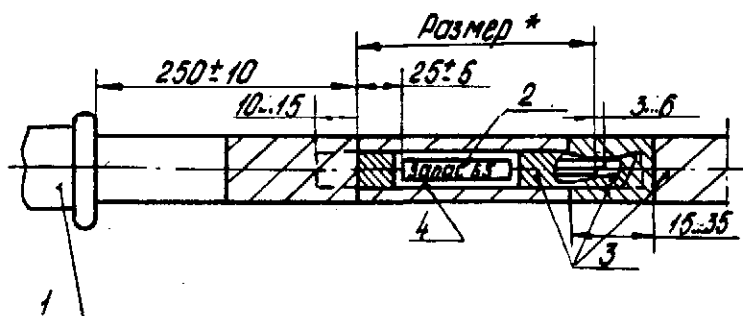
Заделка запасных проводов у разъема
