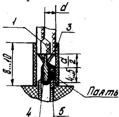
а) без перемычки
