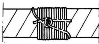
Вязка широкого бандаж шириной свыше 10 мм
