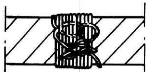
Вязка узкого бандаж шириной от 5 до 10 мм
